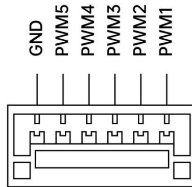
PWM
