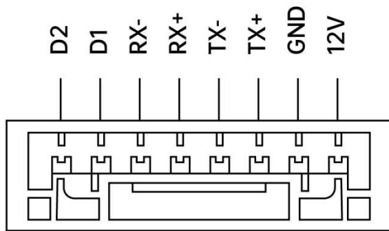
LAN1 & LAN2
